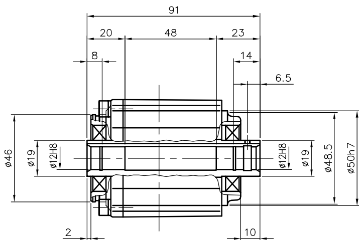
出力軸部詳細
