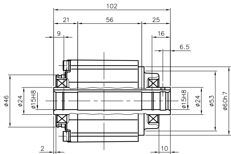
出力軸部詳細
