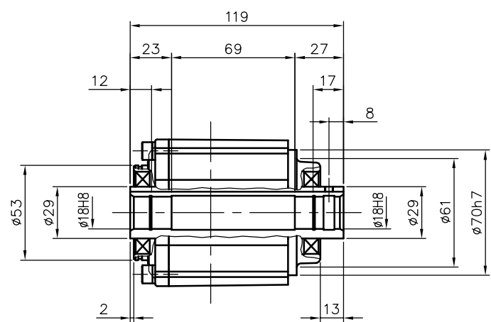
出力軸部詳細
