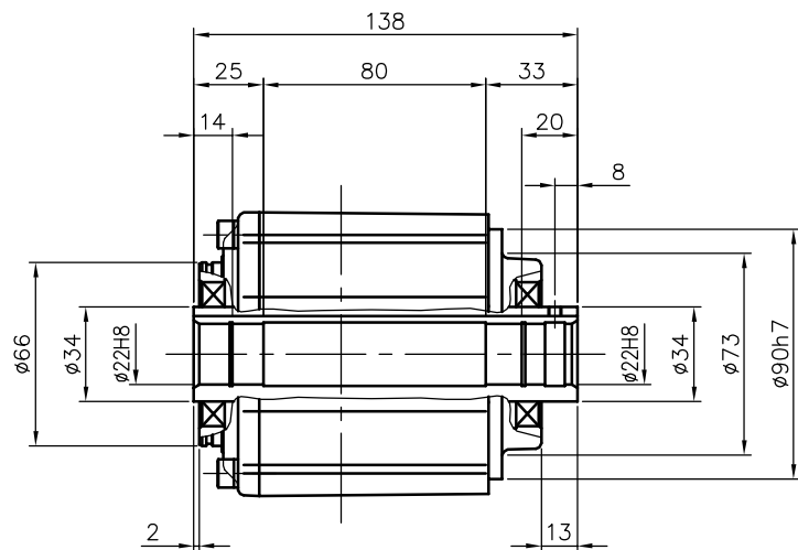
出力軸部詳細
