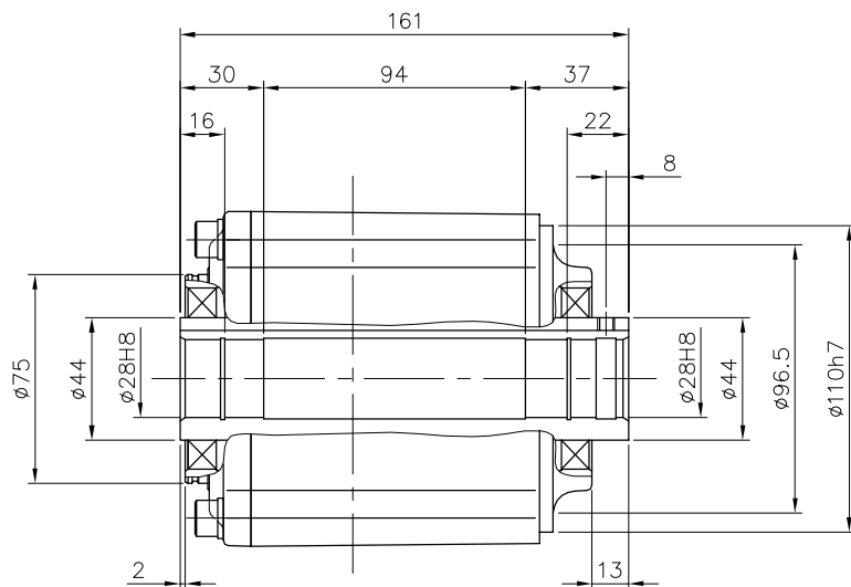
出力軸部詳細
