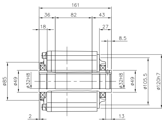
出力軸部詳細
