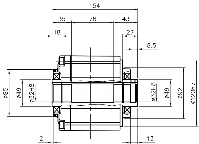
出力軸部詳細
