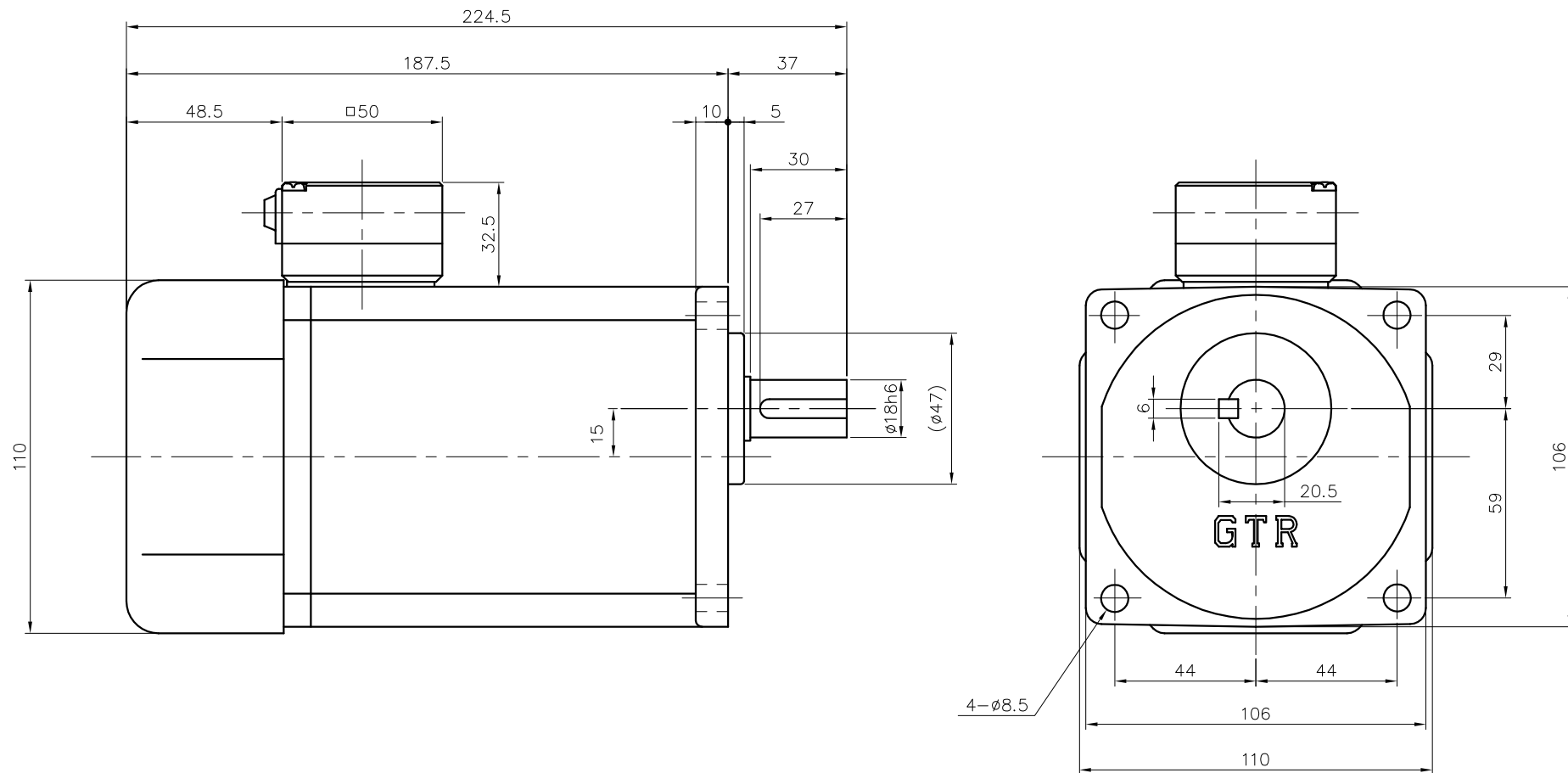
モータ仕様
