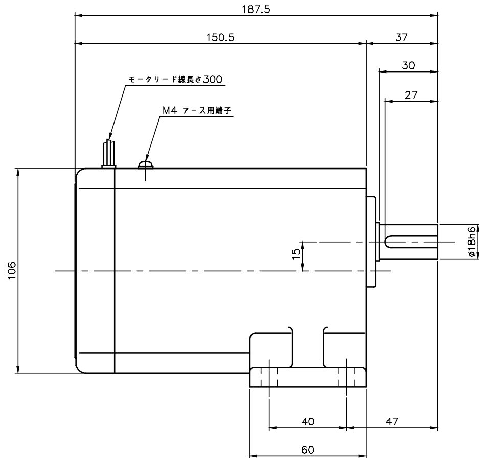
モータ仕様
