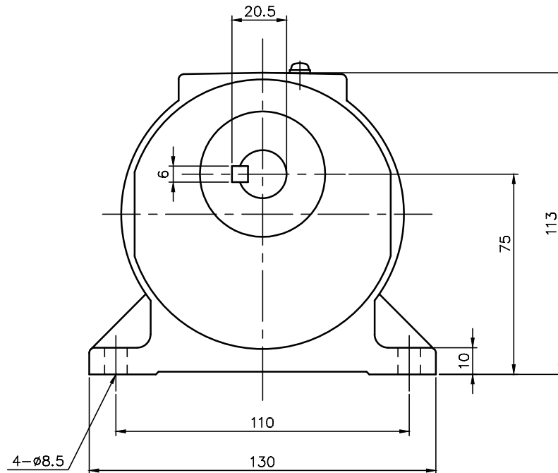
減速機仕様
