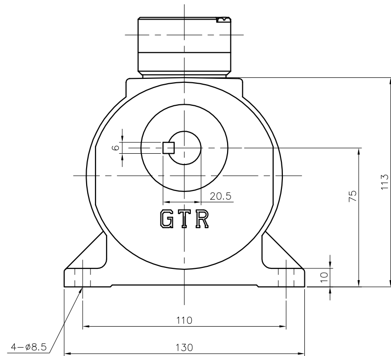
減速機仕様
