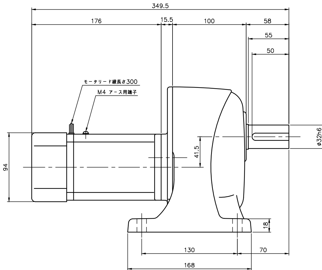
モータ仕様
