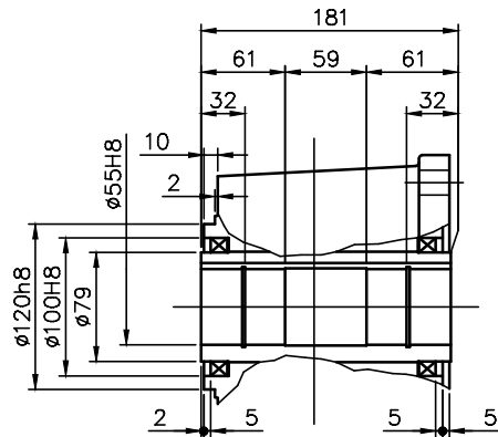
出力軸部詳細
